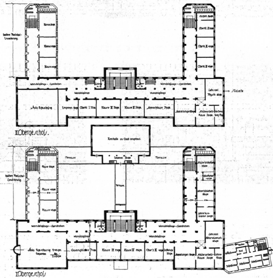
Abb. 64 u. 65. GRUNDRISS.
