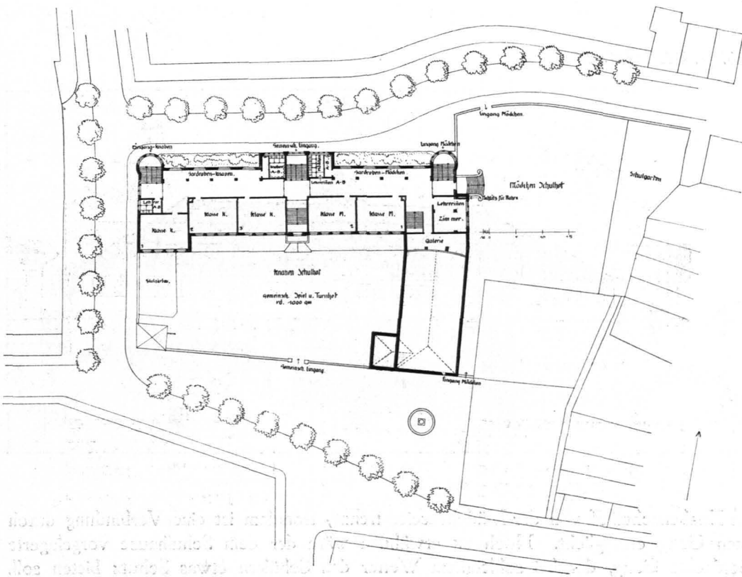
Abb. 50. ERDGESCHOSS. (M. 1 : 1000.)
