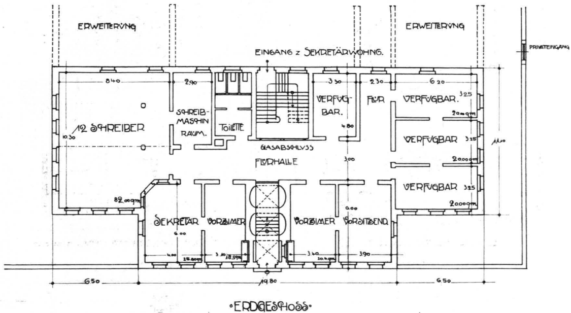
Abb. 47. GRUNDRISS. (M. 1:300.)
