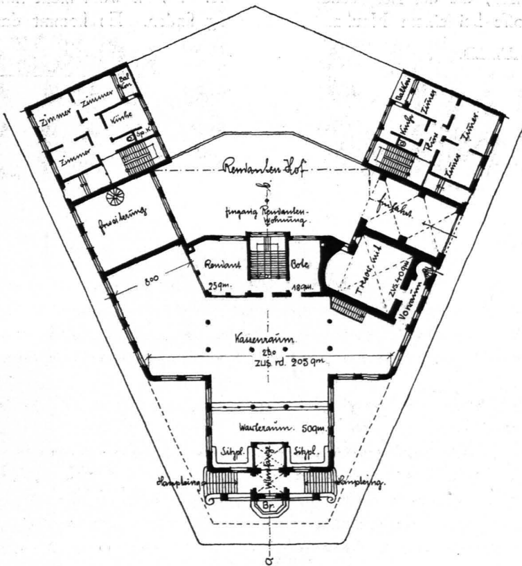
Abb. 41. ERDGESCHOSS. (M. 1:500.)
