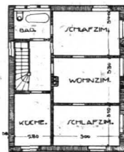
OBERGECHOSS.
