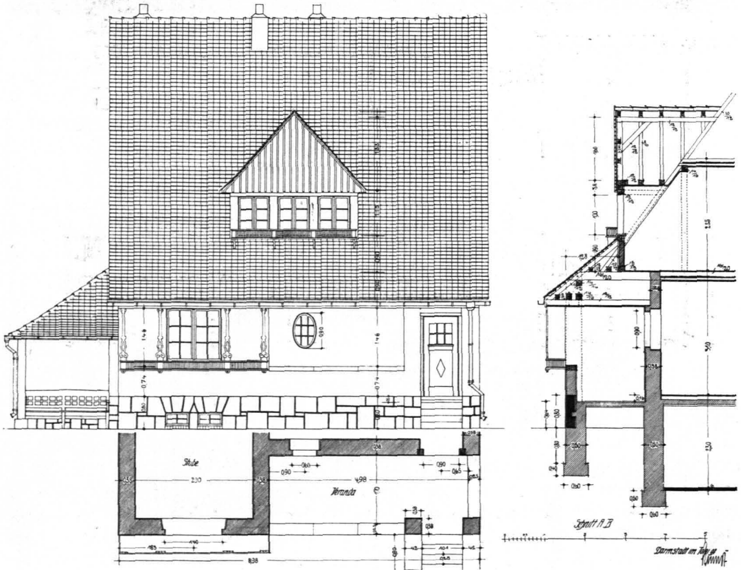
Abb. 19. WESTANSICHT. (M. 1:115.)
