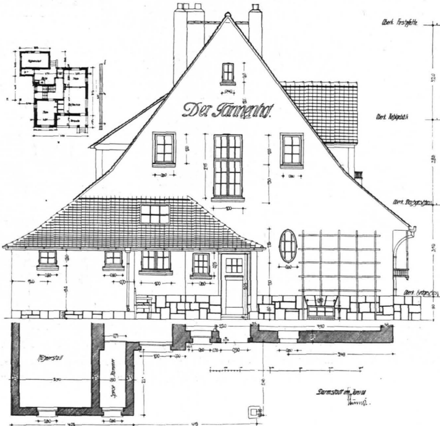
Abb. 17. NORDANSICHT.
