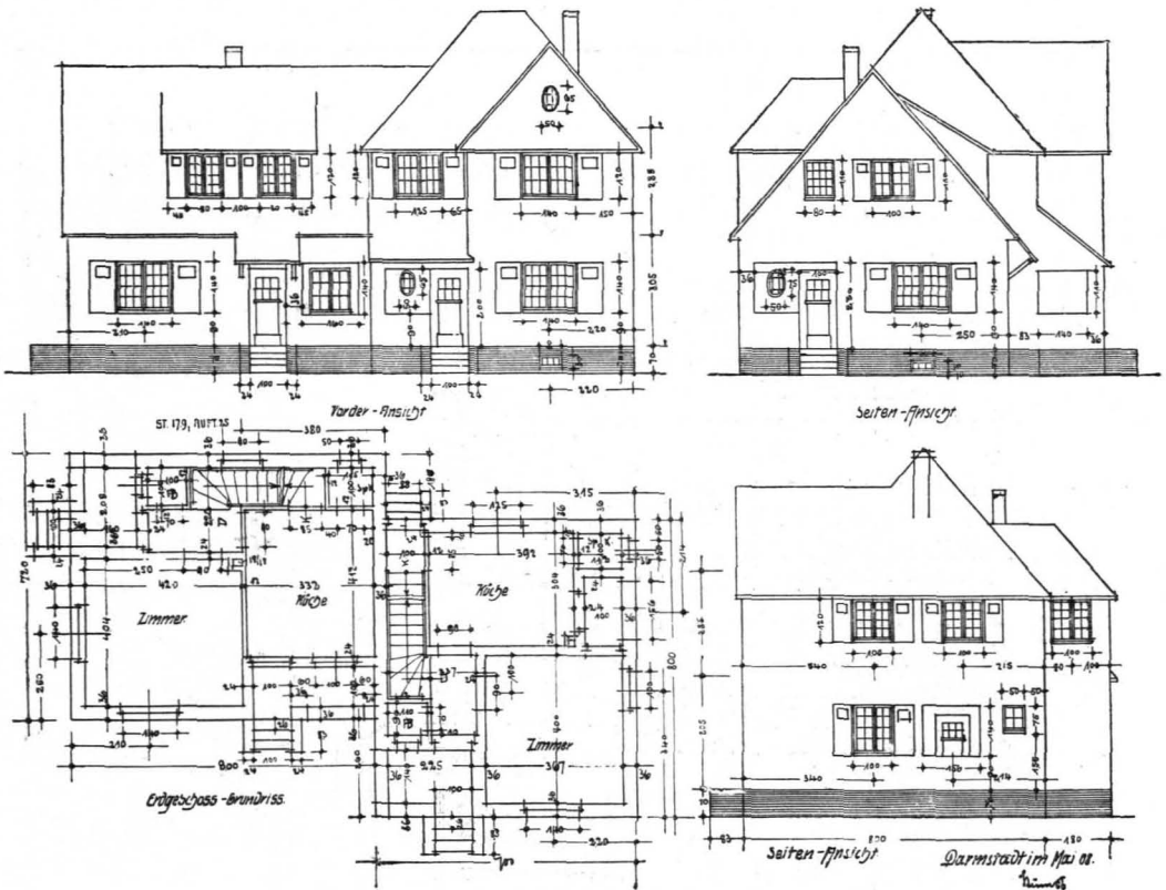
Abb. 7. VORDERANSICHT. (M. 1:125).
