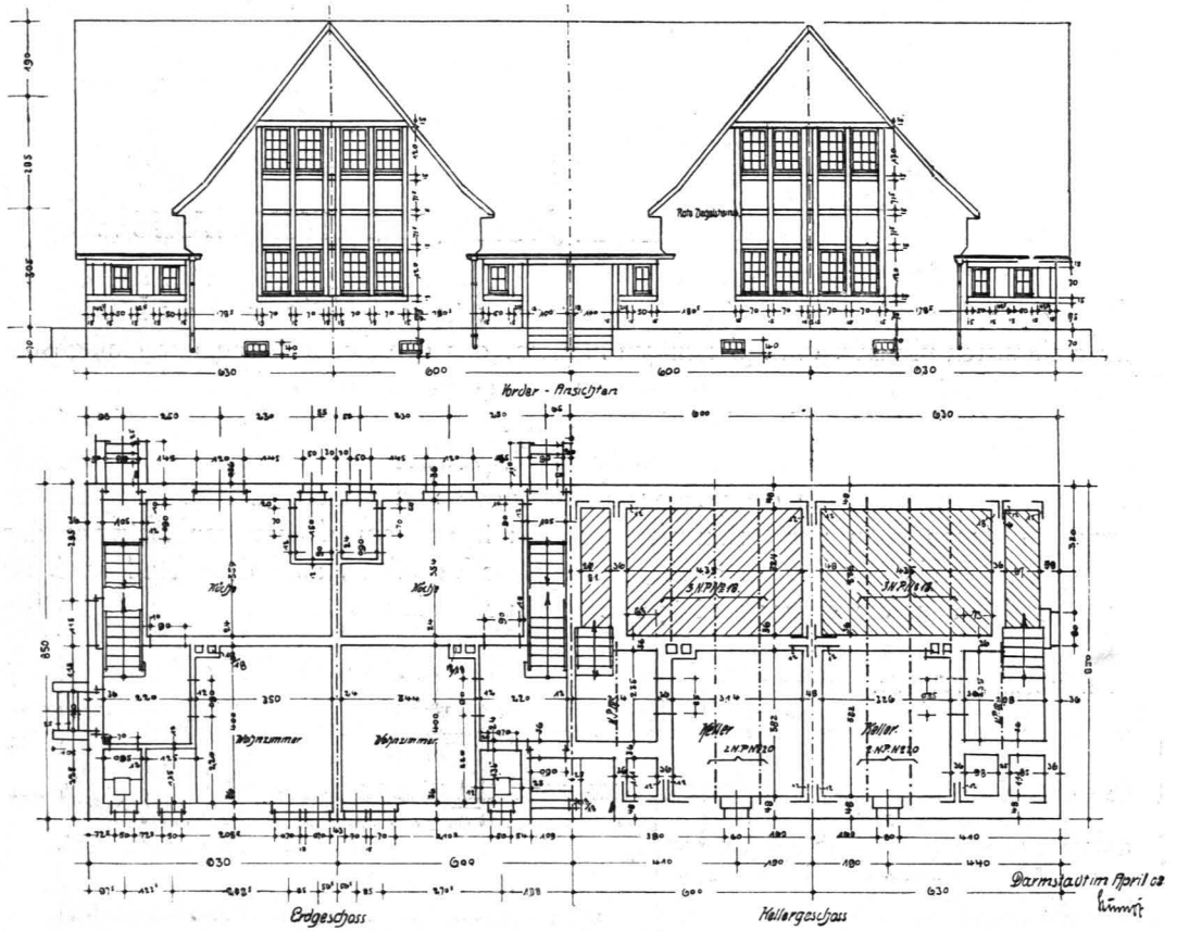
Abb. 2. ANSICHT UND GRUNDRISS. (M. 1:200.)
