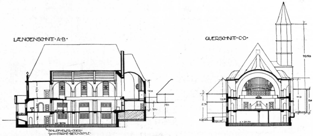
Abb. 155. LÄNGEN- UND QUERSCHNITT.
