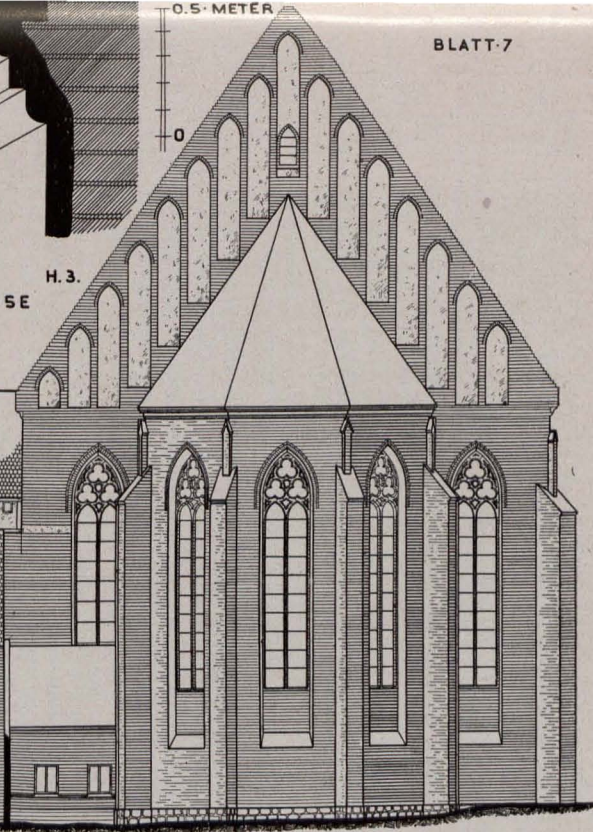
OSTANSICHT
