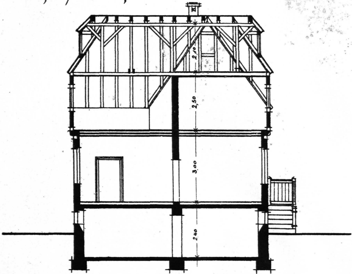
Quer-Schnitt.
