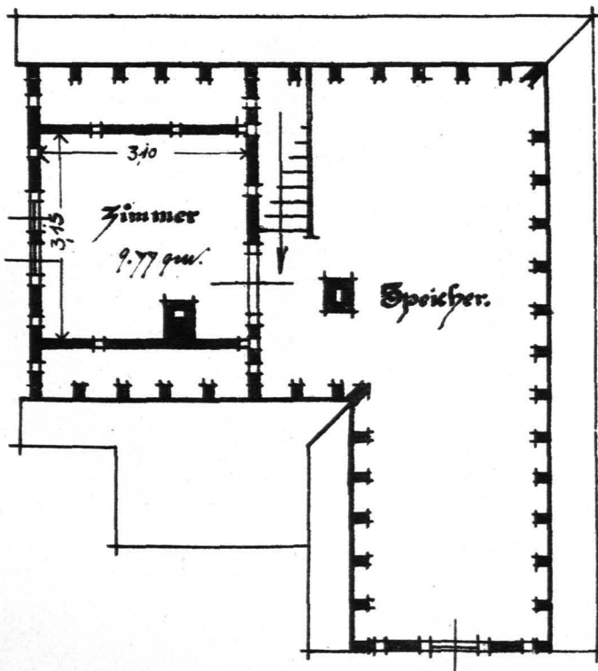
Dachgeschoss.
