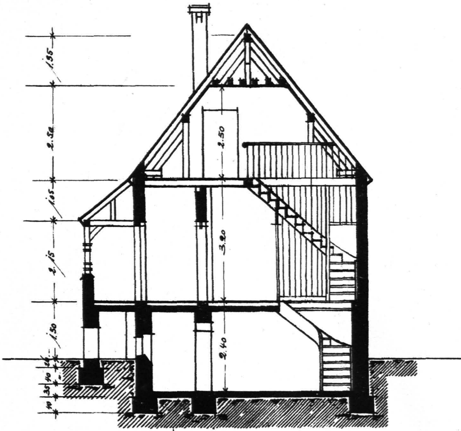
Quer. Schnitt.
