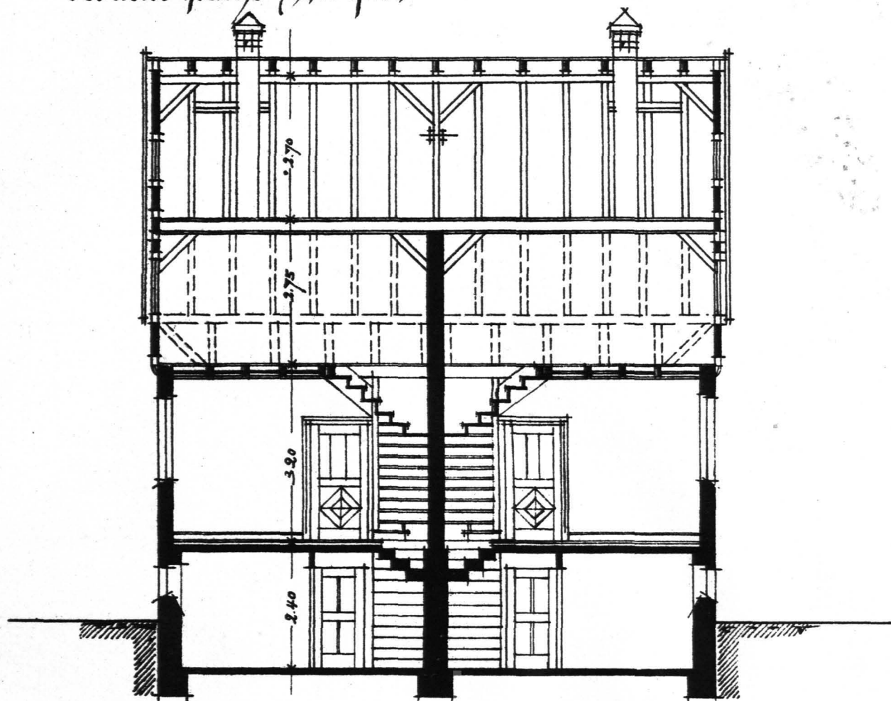
Quer-Schnitt,
