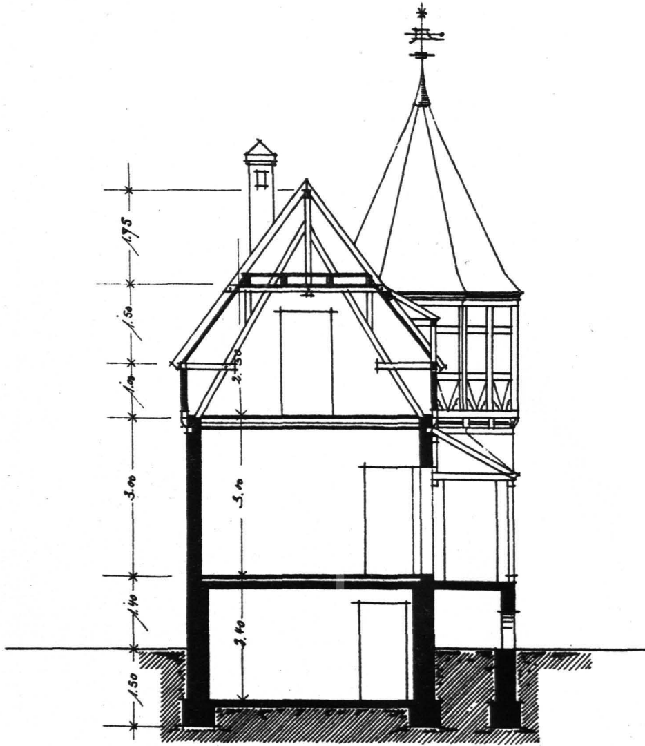
Quer-Schnitt.
