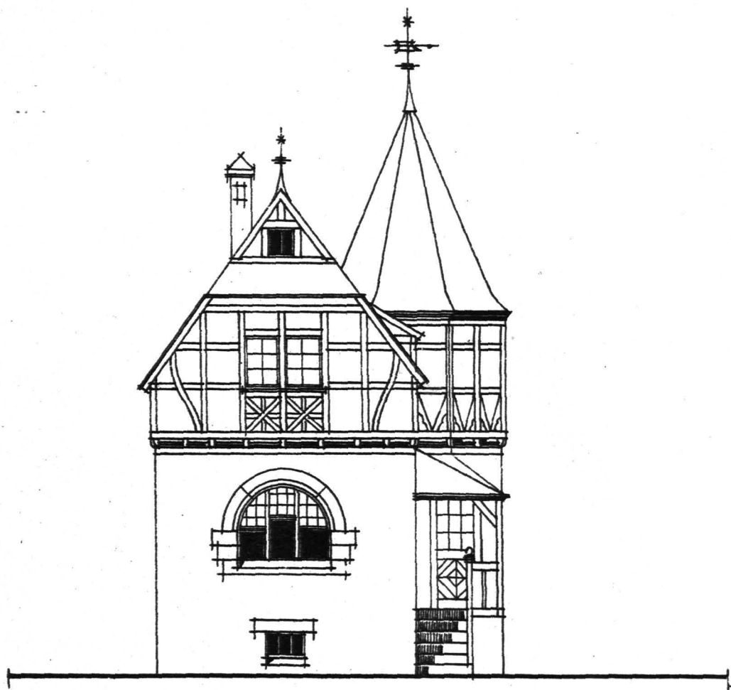
Seiten-Ansicht.
