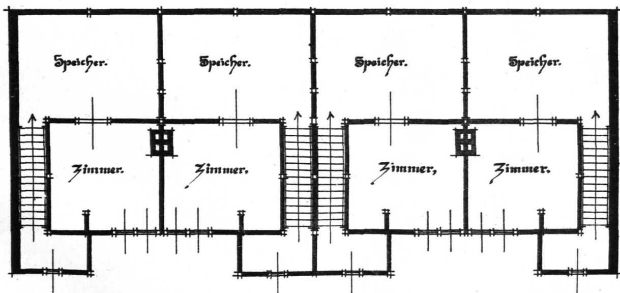
Dachgeschoss.
