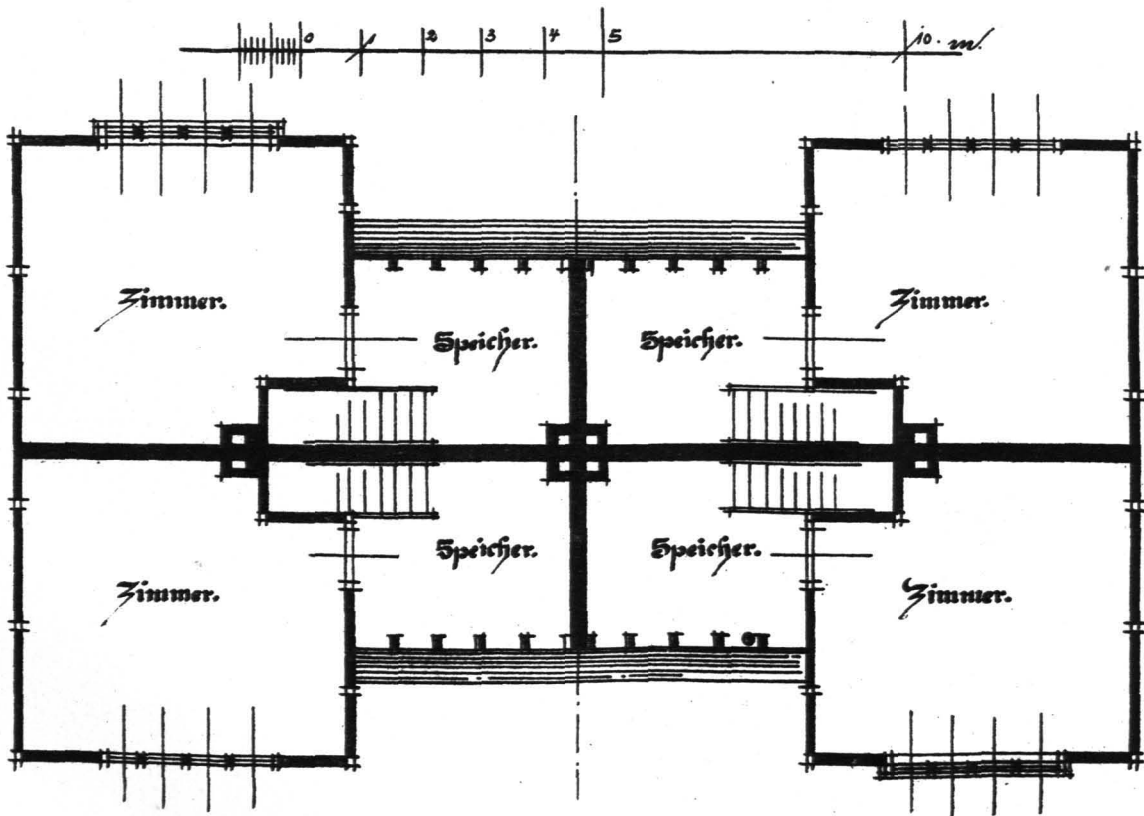
Dachgeschoss.
