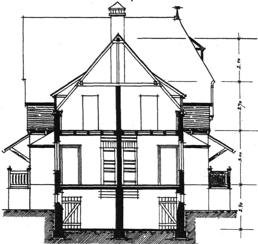
Guer-Schnitt,
