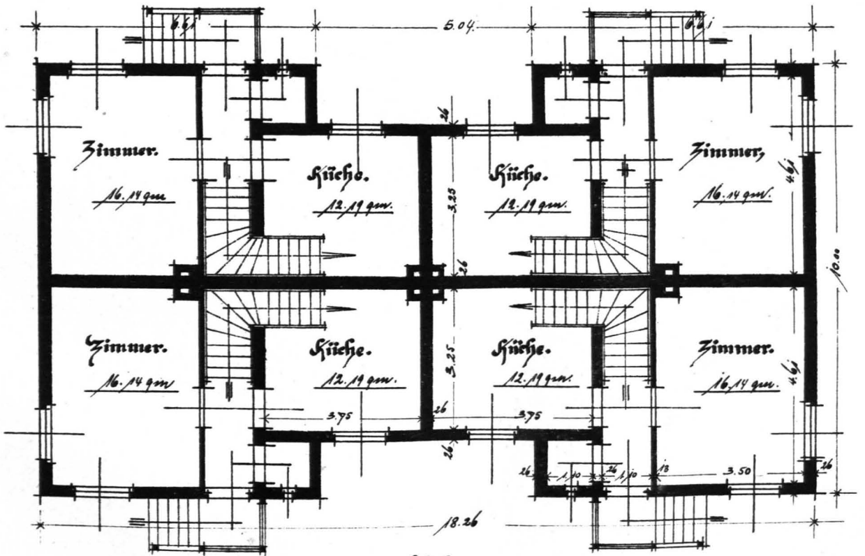
Erdgeschoss,
