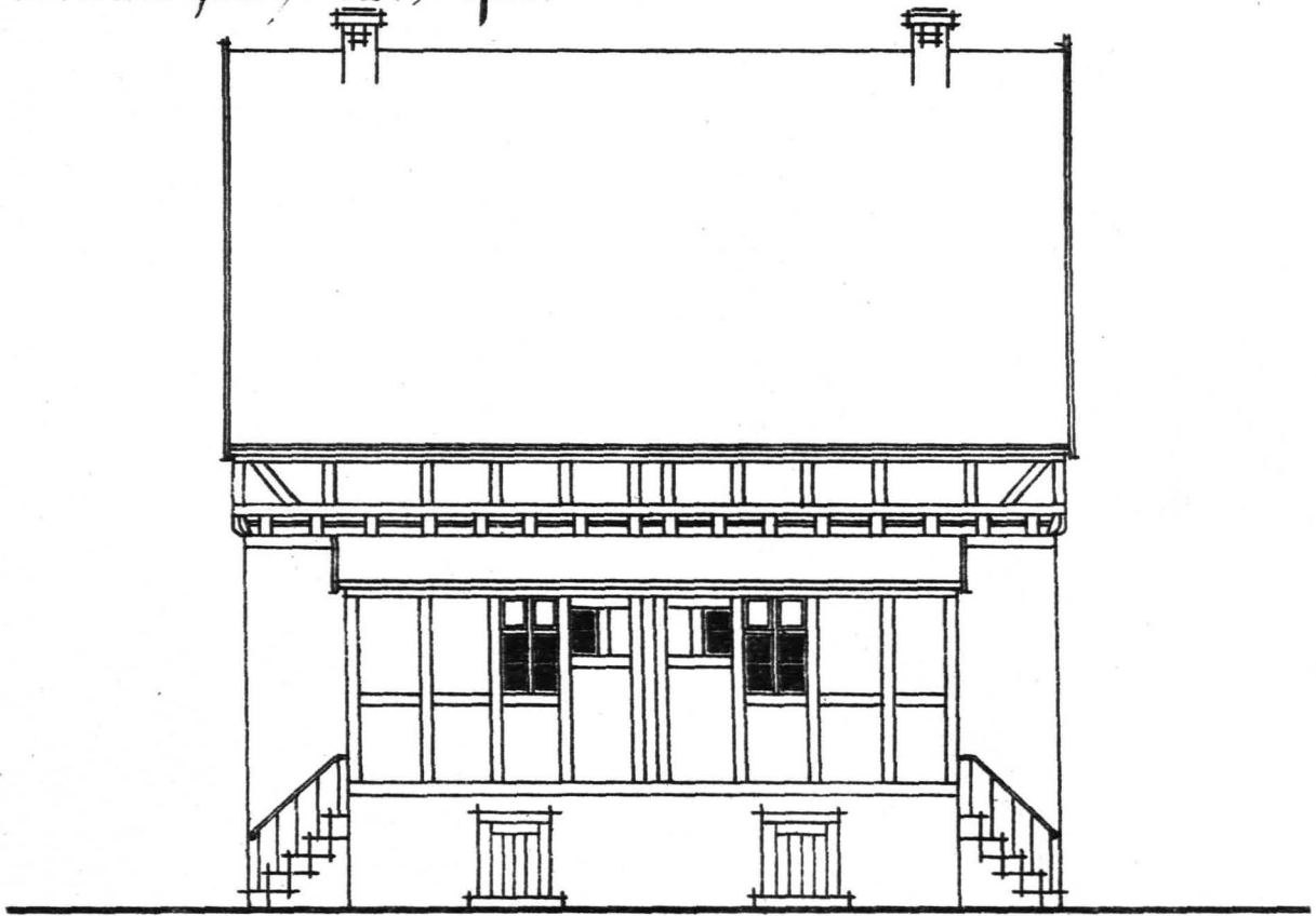
Hinter-Ansicht.
