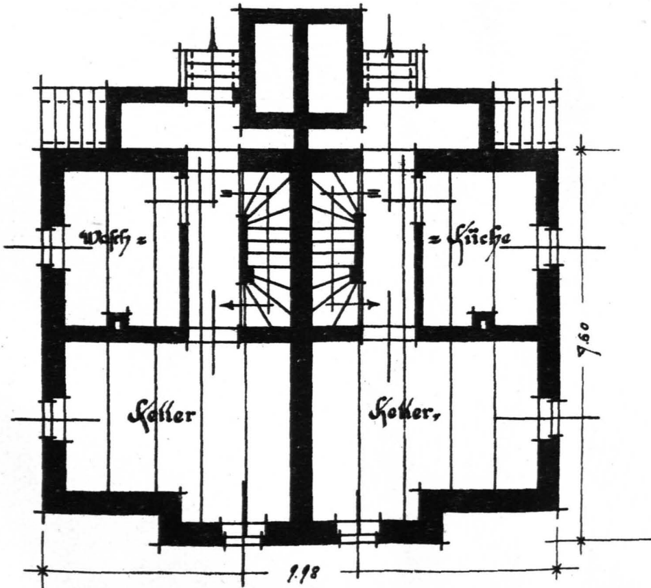
Kellergeschoss.
