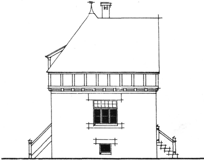
Seiten-Ansicht,
