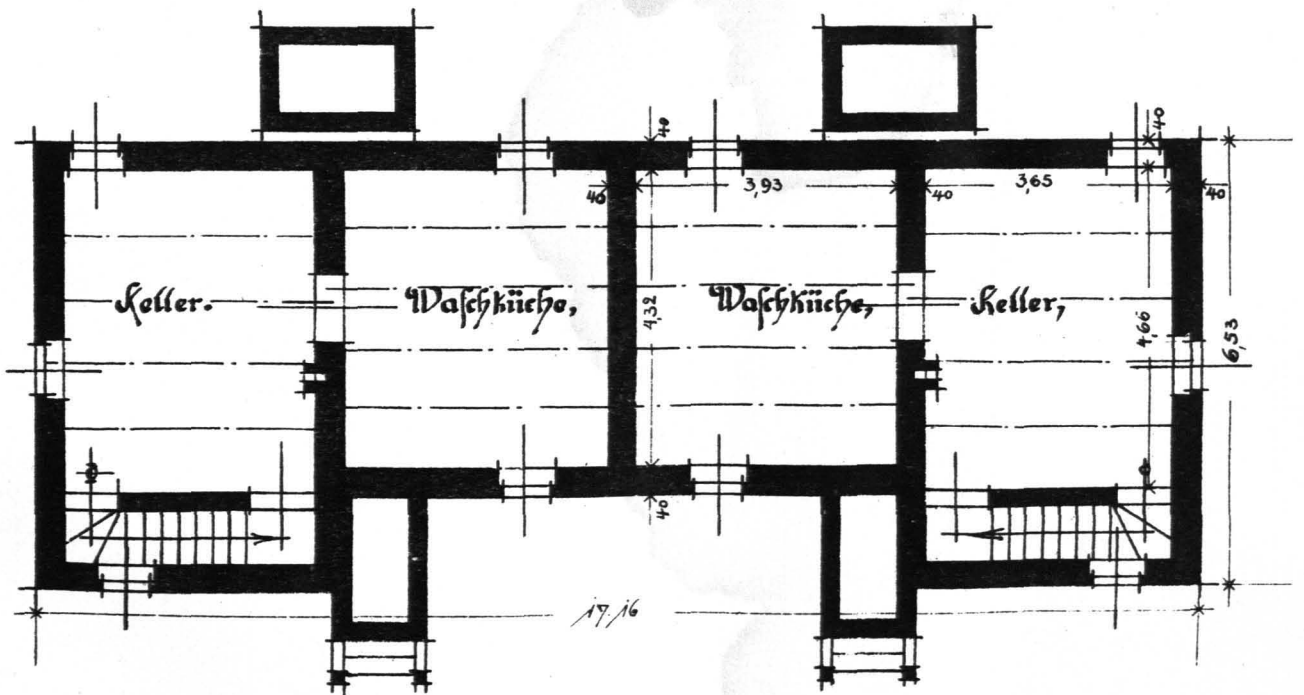
Kellergeschoss,
