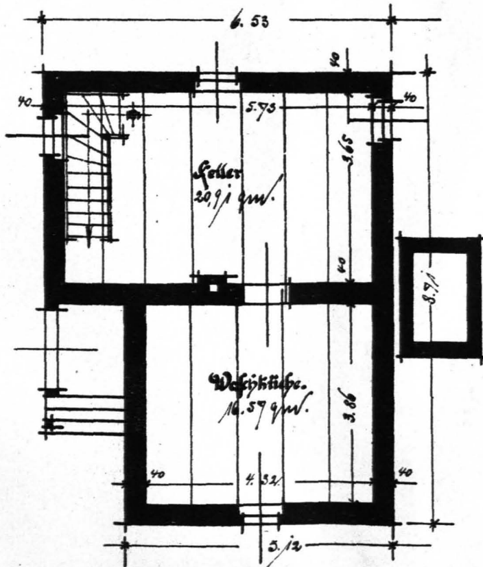
Kellergeschoß.
