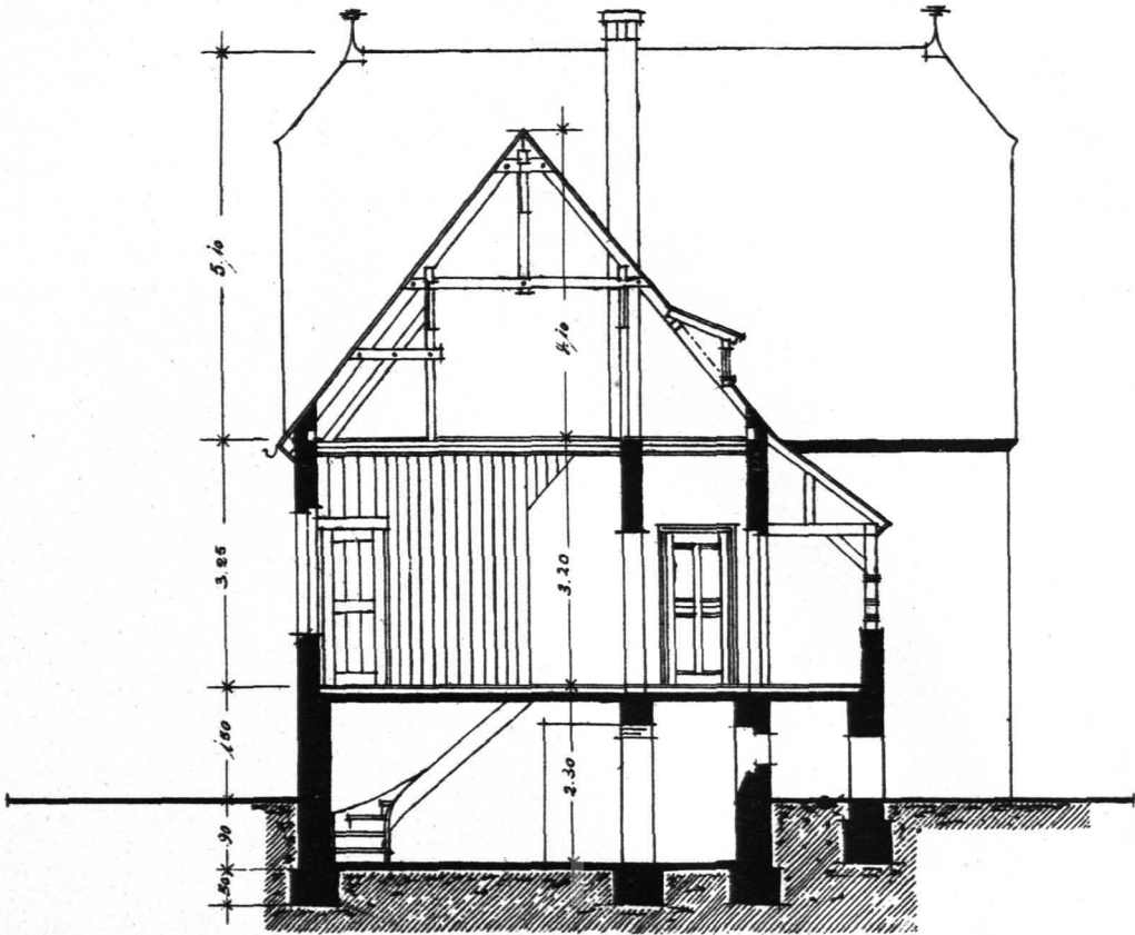
Quer-Schnitt.
