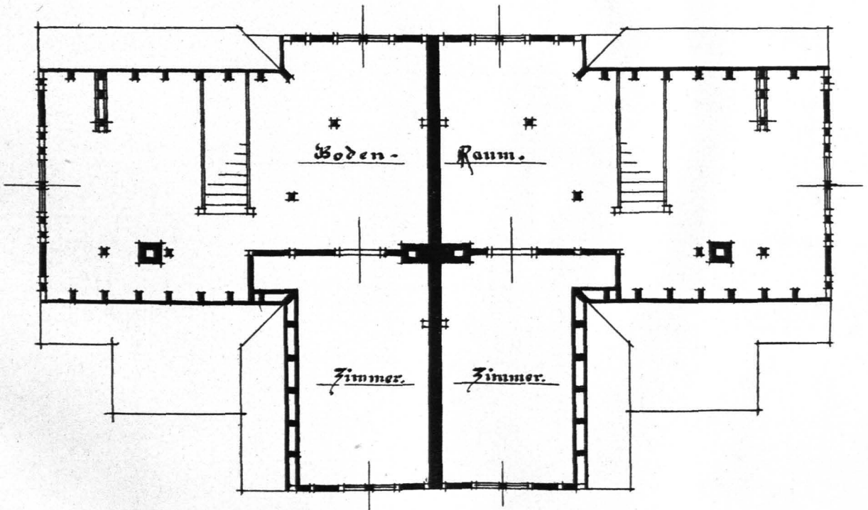
Wachgeschosz.
