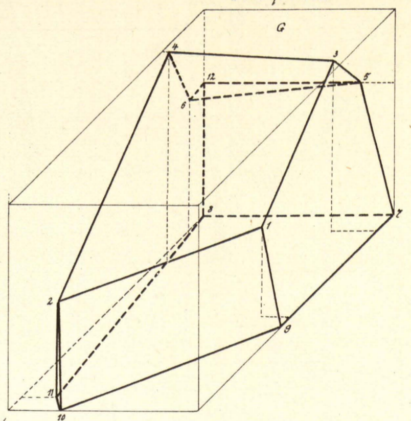
Stirndeckquader
