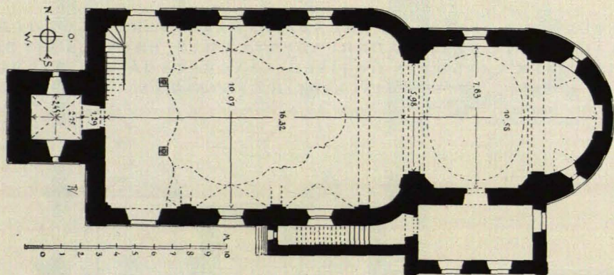
HETZENBACH (VGL. S. 67). GRUNDRISS DER KIRCHE, 1764
