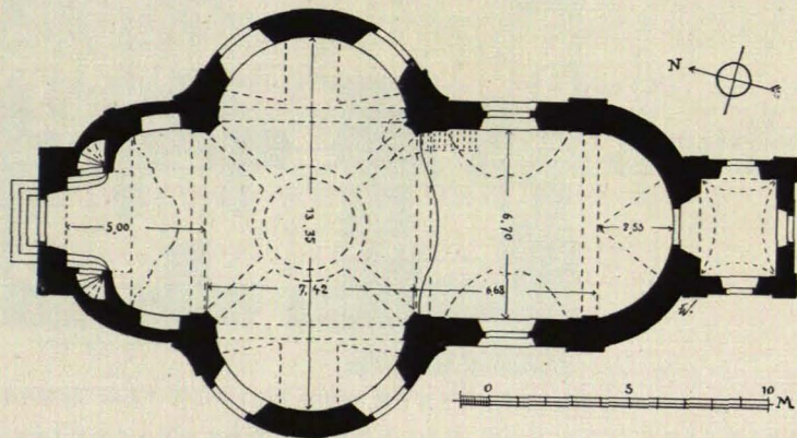
MARCHANEY (VGL. S. 67). GRUNDRISS DER KIRCHE, 1755
