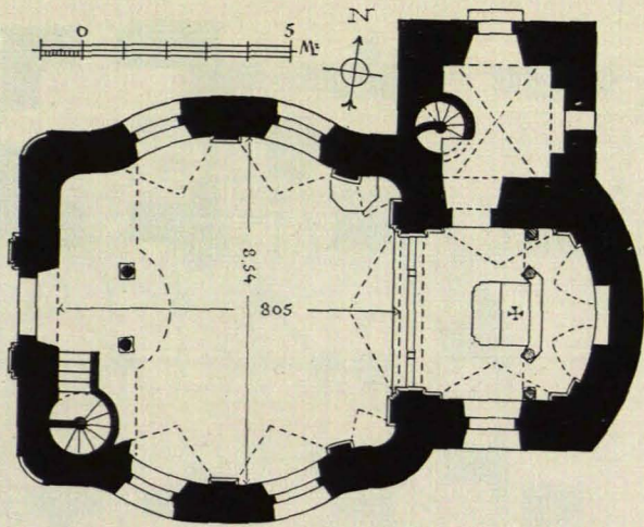
SIMBACH (B.-A. BEILNGRIES). GRUNDRISS DER KAPELLE, VON JOH. JAKOB BERG UM 1763
