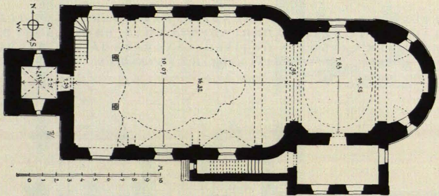
HETZENBACH (VGL. S. 67). GRUNDRISS DER KIRCHE, 1764
