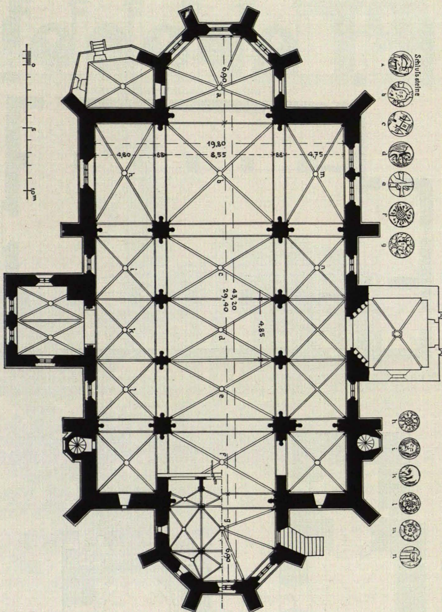
NABBURG. GRUNDRISS DER PFARRKIRCHE (VGL. S. 88)
