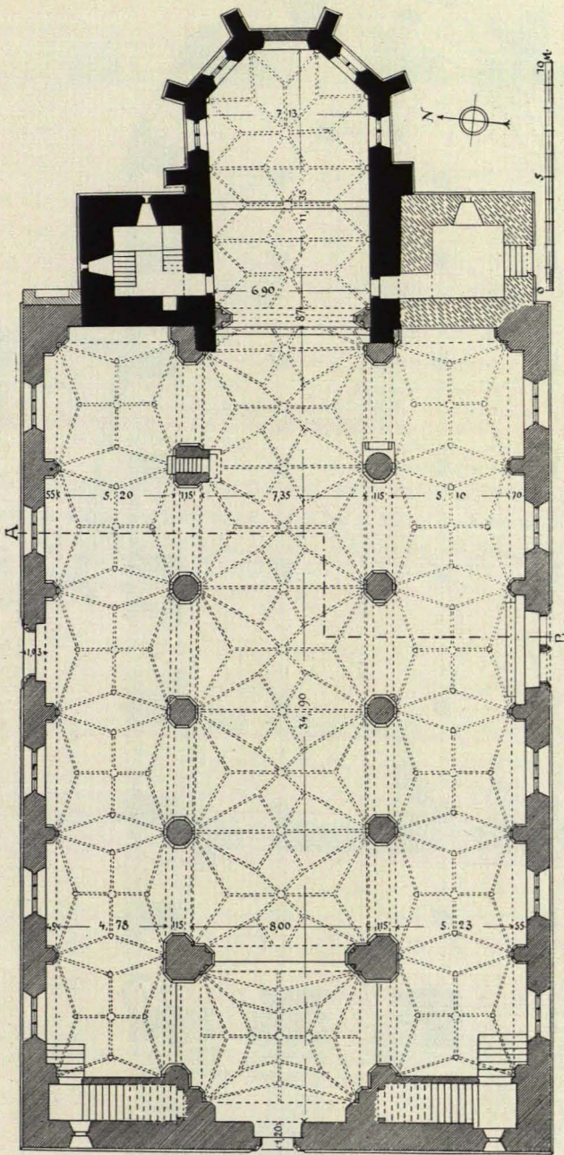
CHAMMÜNSTER. GRUNDRISS DER PFARRKIRCHE (VGL. S. 22)
