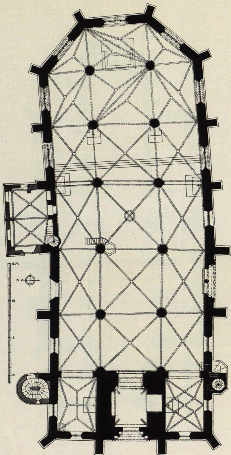
NEUMARKT. GRUNDRISS DER PFARRKIRCHE (VGL. S. 25)
