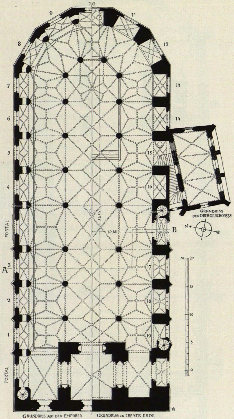
AMBERG. GRUNDRISS DER MARTINSKIRCHE (VGL. S. 56)
