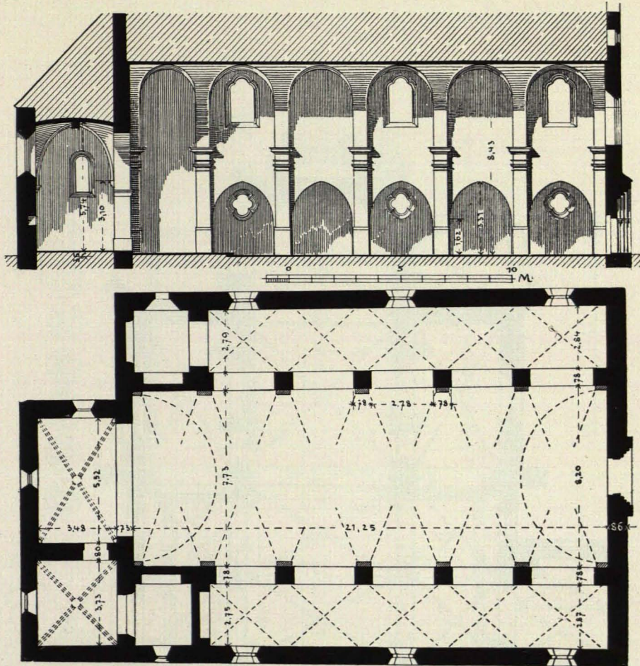
PERSCHEN (B.-A. NABBURG). GRUNDRISS UND LÄNGSSCHNITT DER KIRCHE (VGL. S. 2)
