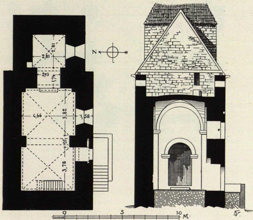
AICHOLDING (B.-A. RIEDENBURG). GRUNDRISS UND QUERSCHNITT DER ROMANISCHEN KIRCHE (VGL. S. 14)
