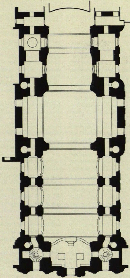
Plan der Kirche.
