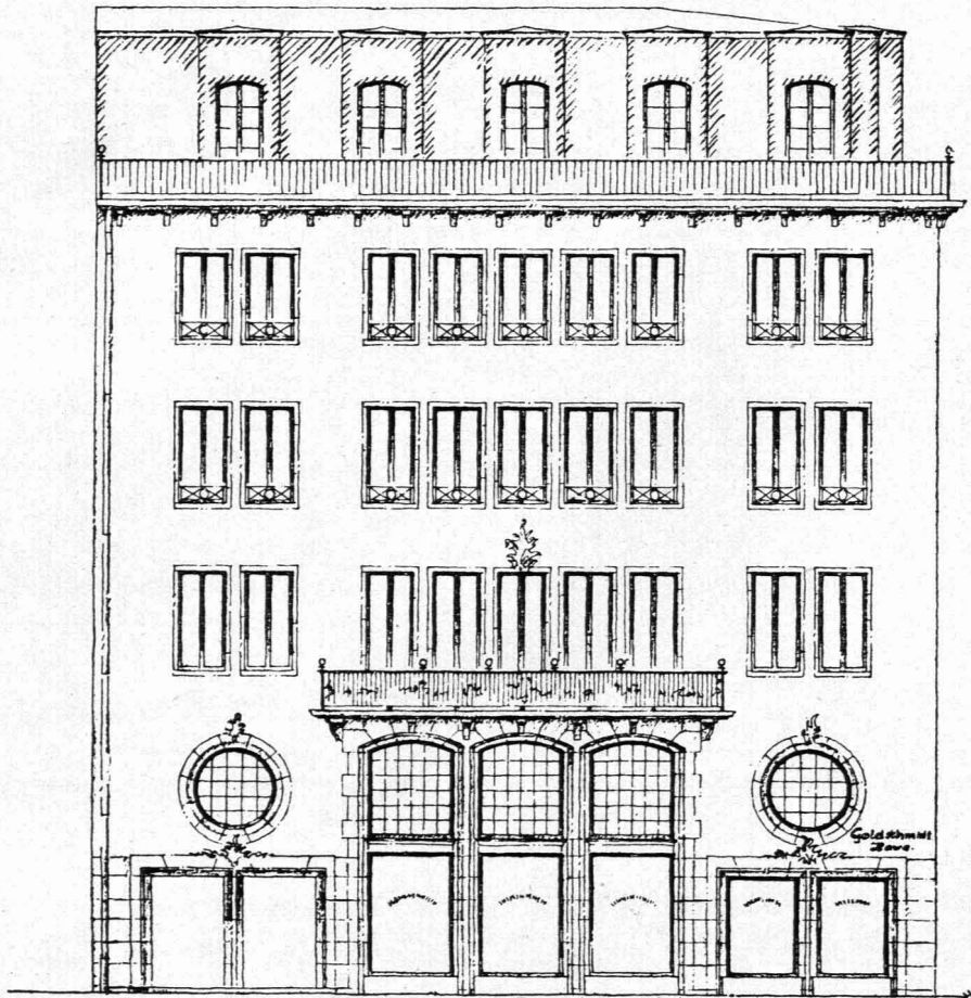
KÖLN / 489 / COLOGNE Fassadenentwurf (vgl. Abb. 491) Design for façade. (Compare Ill. 491) Arch : Paul Bonatz
