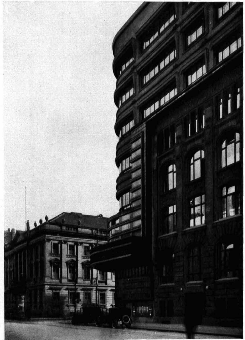
424 / BERLIN Mossehaus. Ein altes Haus überbaut durch einen Neubau An old publishing house (Jerusalener Str.) built over by new addition (Compare Ill. 443) Arch.: Erich Mendelsohn
