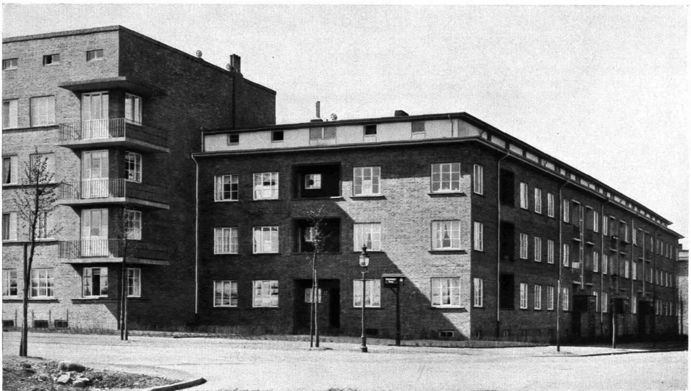
344-45 / HAMBURG - BARMBECK Kleinwohnungen Small Flats Arch.: Hans und Oskar Gerson
