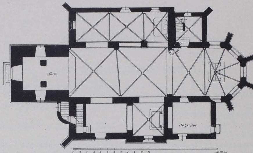
Fig. 31. Alland, Pfarrkirche. 1 : 300 (S. 1).
